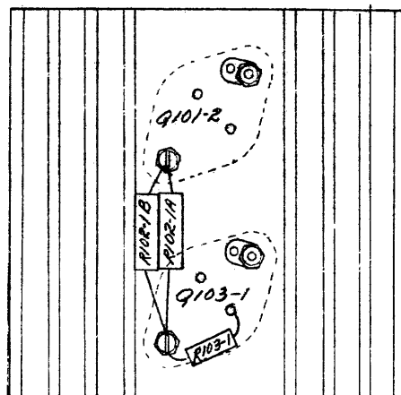
VIEW A-A
